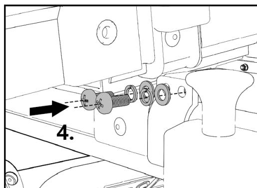
Figura 4: Montaggio dell'attacco sul portabiciclette
