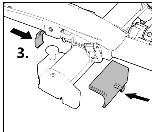
Figura 3: Montaggio dell'attacco sul portabiciclette
