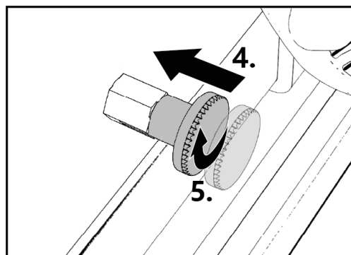
Figura 10: Rimuovere l'estensione
